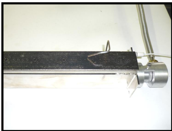
Electrode de contrôle de flamme pour fonctionnement sans veilleuse.
