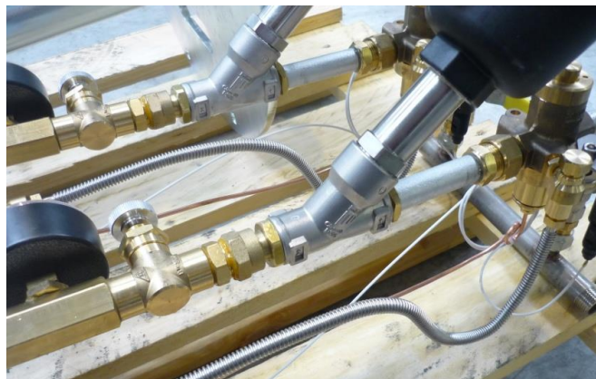
Montage de 2 « flexipipes » : liaisons diam.6mm pour pilote d'allumage fonctionnant à 2bar.
