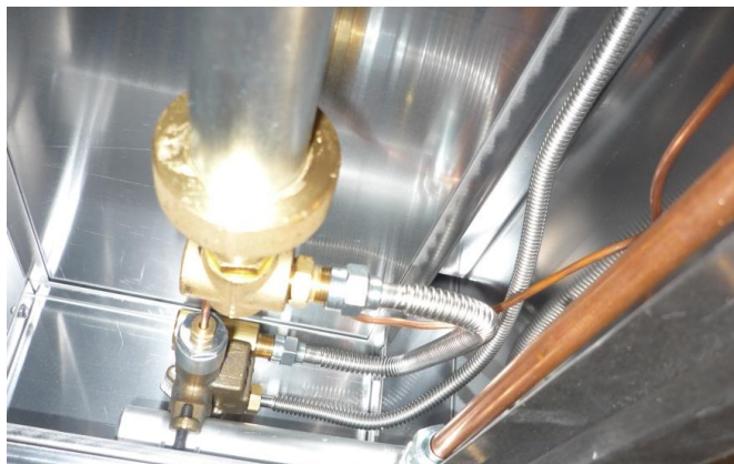
Montage de 2 « flexipipes » : liaisons diam.8mm pour brûleur principal et diam.6mm pour veilleuse.
