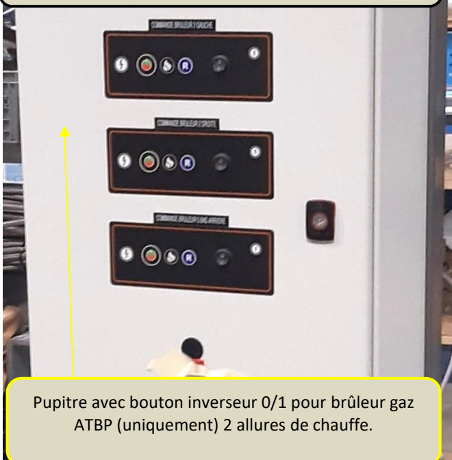
Coffret 400x500 CPG3ATBP à 3 pupitres de commande double allure de chauffe.
